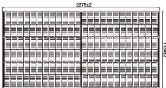
Fig. 3. Dimensiones de módulo fotovoltaico de 550W Jinko Solar.
