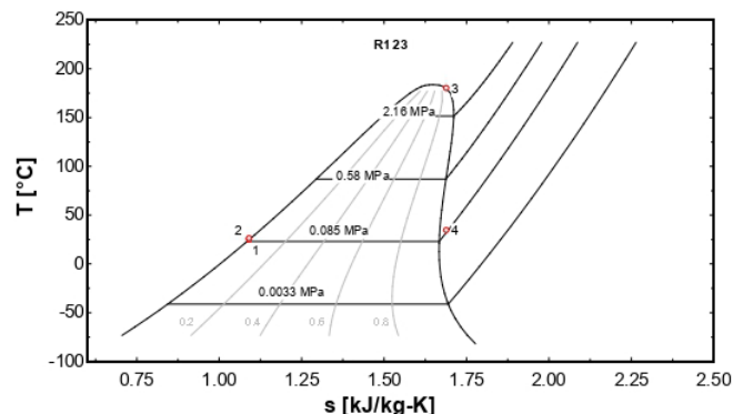
Fig. 5. Diagrama T-s R123
