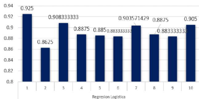
Fig. 4. Exactitud de RL.
