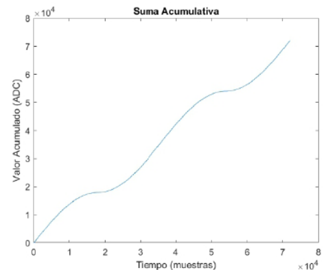
Fig. 4. Curva de la suma acumulativa de un ciclo de la función seno.
